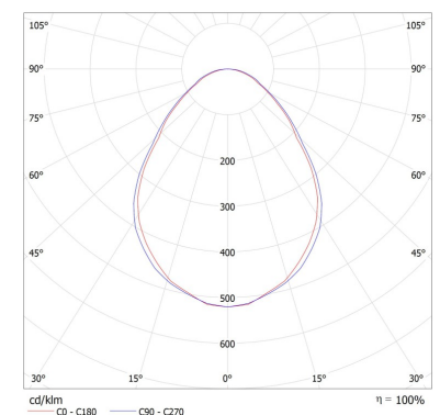
Lichtstärkeverteilung: (Polar)
